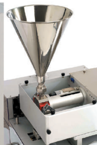
Dosatore semi automatico per corpi solidi; MP 100 con dosatore polveri; Dosatore liquidi; Dosatore creme Semi automatic solid bodies doser; MP 100 with powder doser; Liquid doser; Cream doser
