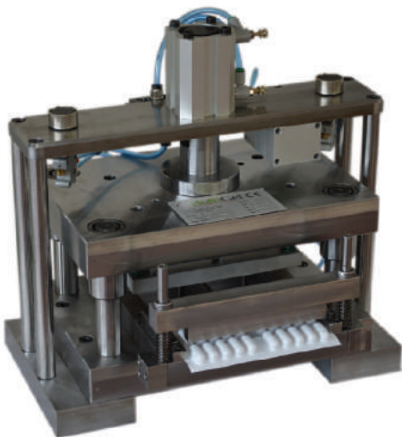
Tranciatore per blister Shearer for blisters
